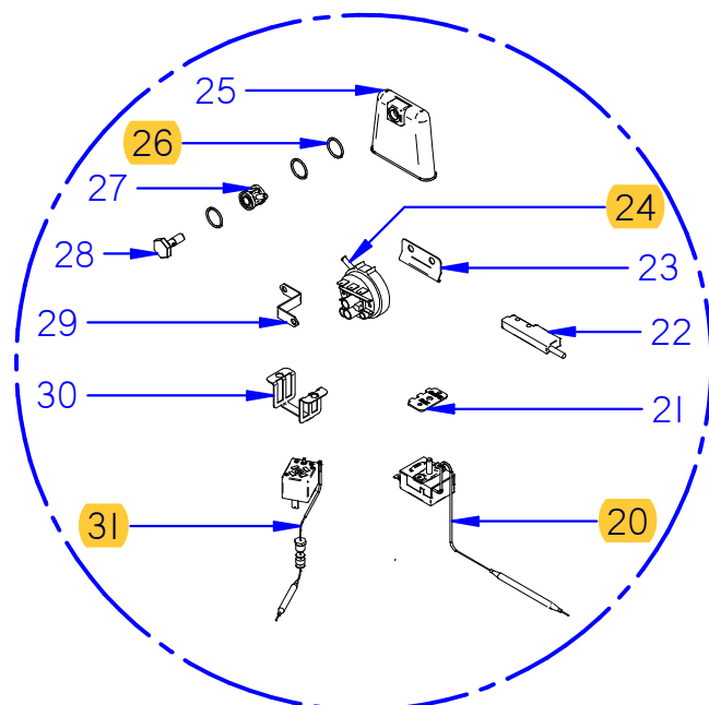
DETALLE B
