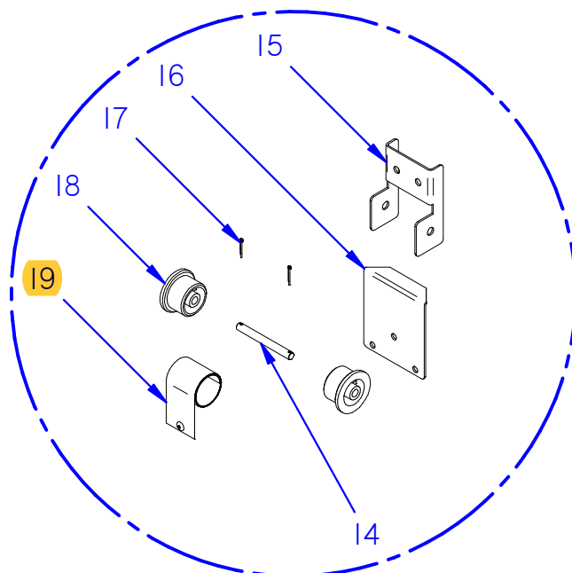
DETALLE A
